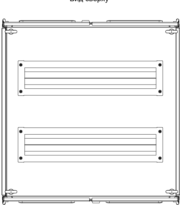
Вид сверху
