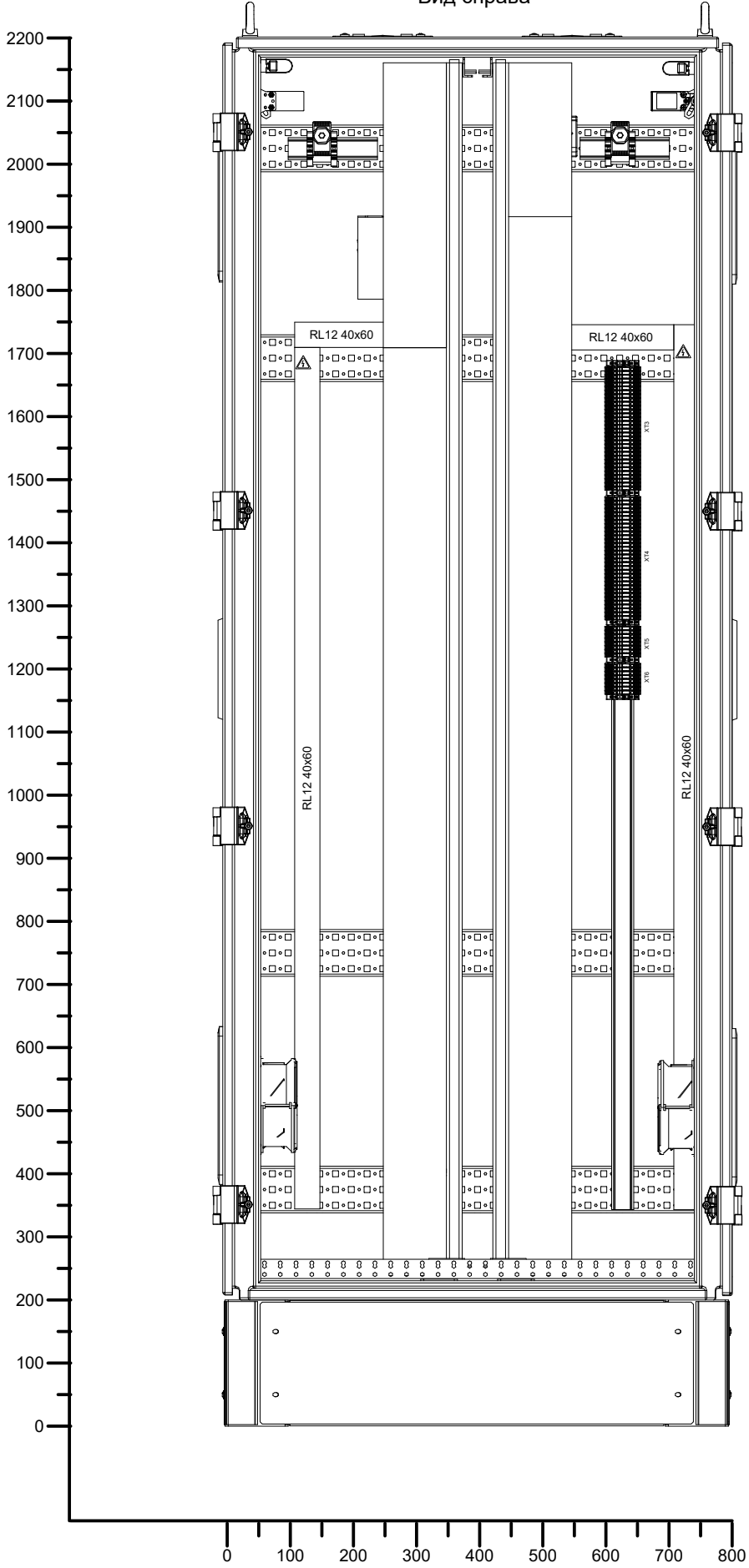
Вид справа
